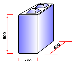
TYPE A4 (gew: 610 kG)
