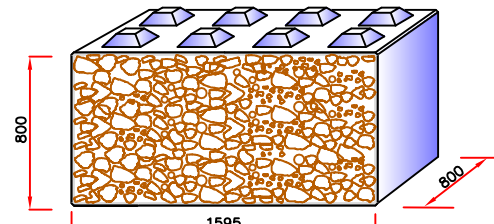
TYPE A1R (gew: 2400 kG)
