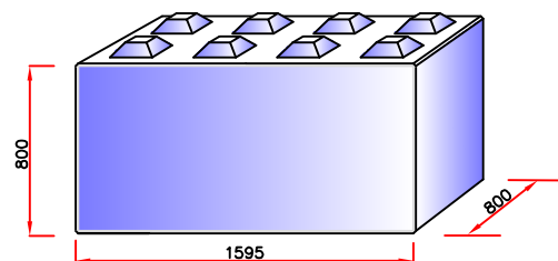
TYPE A1 (gew: 2400 kG)
