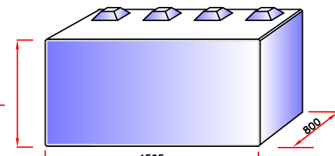
TYPE A1H (gew: 2375 kG)
