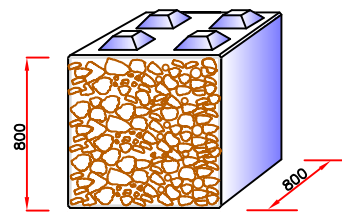
TYPE A2R (gew: 1250 kG)
